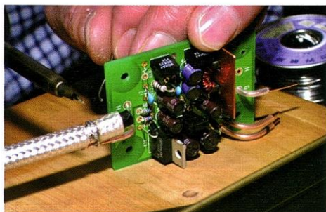
基板を取り外し、別に用意した同軸ケーブルを2本ハンダ付けする
