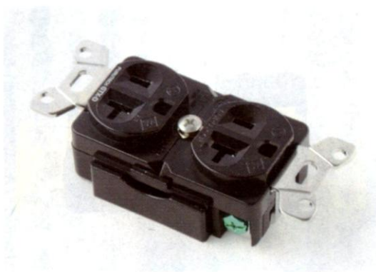
フルテック GTX-D (R) (¥17,640)。GTX Series のハイエンドグレード壁コンセント (20A 125V)、純銅のロジウムメッキ仕様。取り付け金具は 2mm の厚みを持つステンレス
