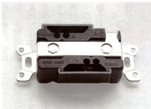
フルテック GTX-D (R) (¥17,640)。GTX Series のハイエンドグレード壁コンセント (20A 125V)、純銅のロジウムメッキ仕様。取り付け金具は 2mm の厚みを持つステンレス
